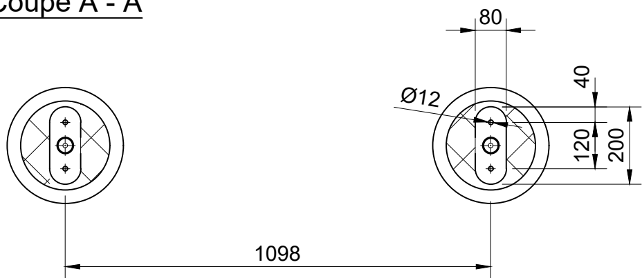
Coupe A - A
