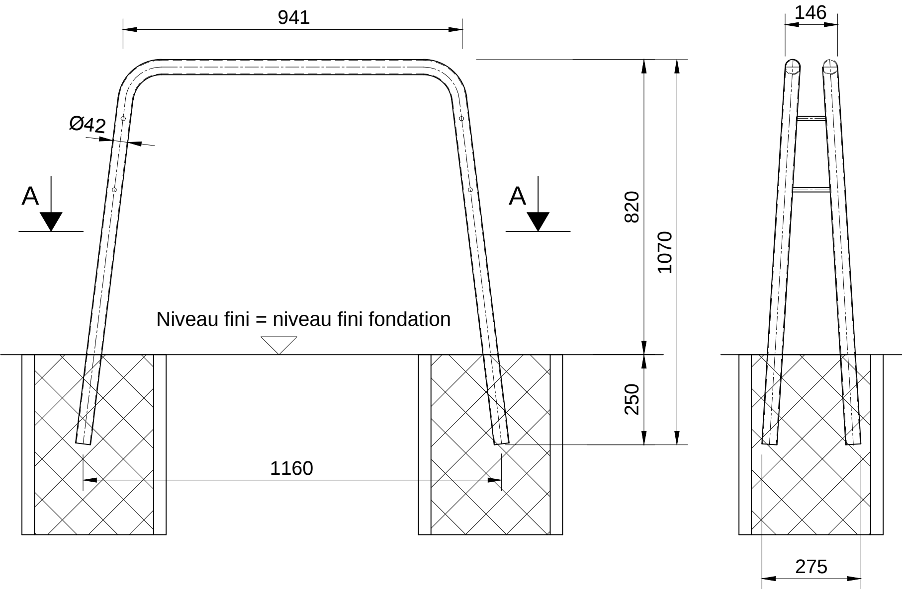
Coupe A - A
