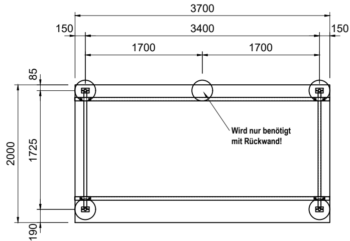
Draufsicht
