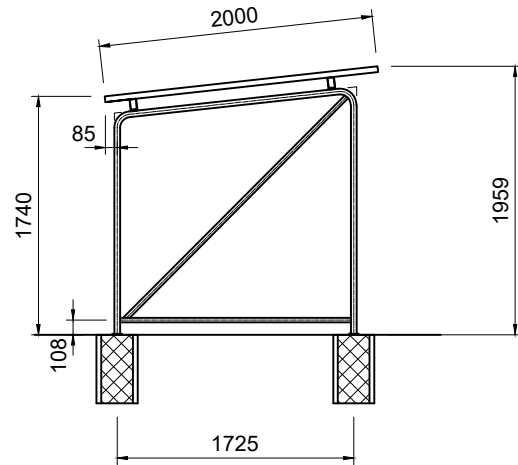
Seitenansicht
