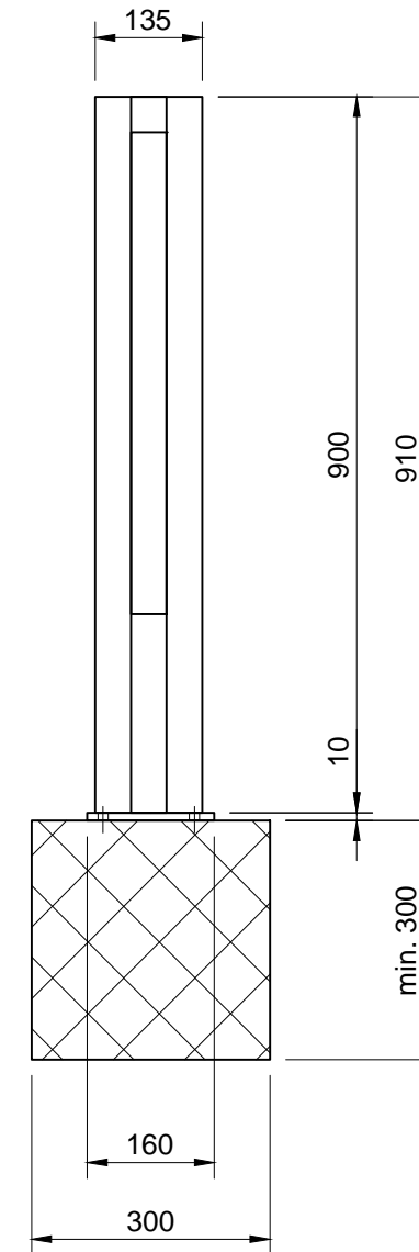
Seitenansicht
