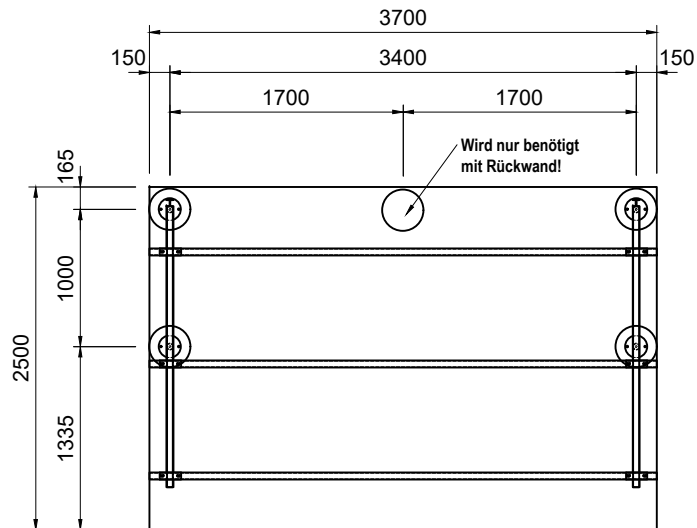
Draufsicht
