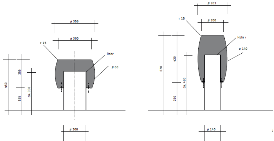
Rubix S1 und Rubix S2 – Sessel und Hocker für längere oder kurze Verweildauer
