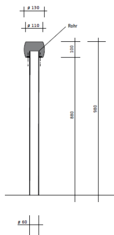
Rubix P1 – Begrenzungspoller fest verankert oder abschliessbar zur Entnahme
