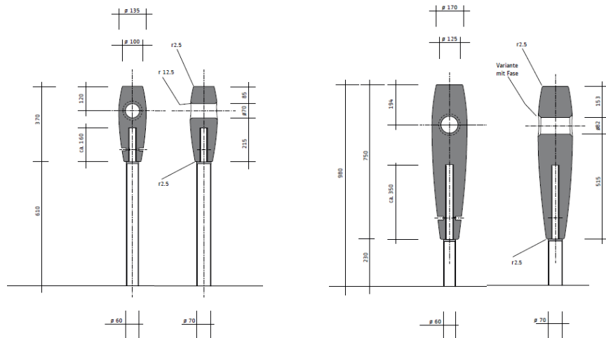
Rubix F1 und Rubix F2 – Velo-Anlehnbügel mit weichen Aufnahmeflächen und Anschliessmöglichkeit
