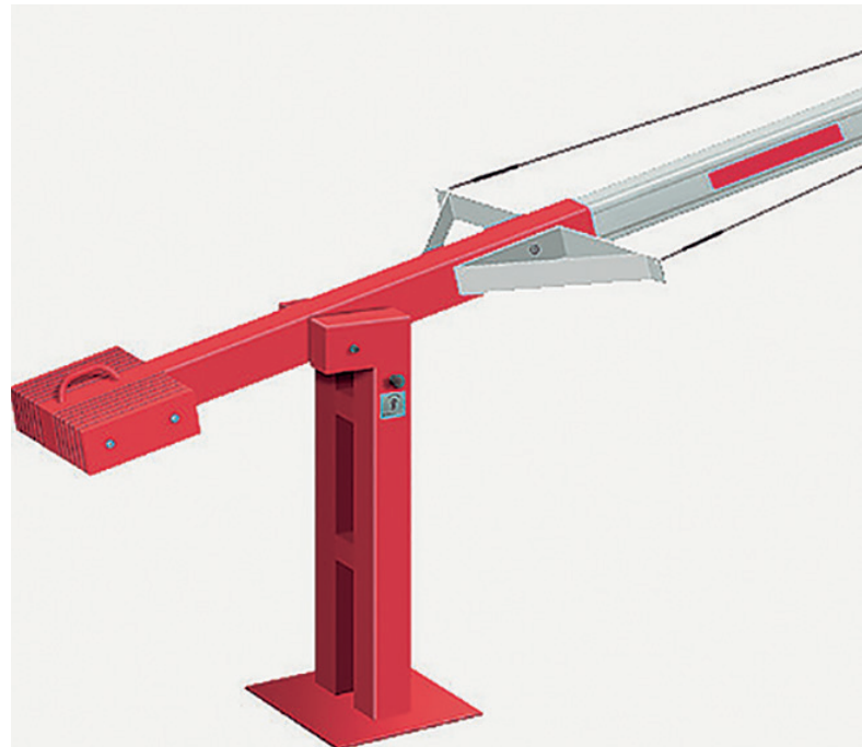
Spezielle Holmabspannung ab Holmlänge 5.50 m
