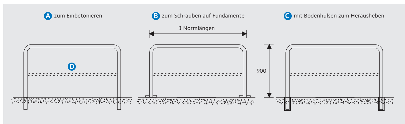
Bodenhülse C mit Vorhängeschloss
