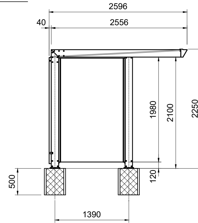
Vue latérale
