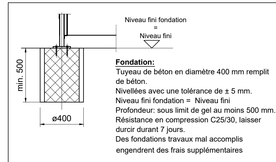
Détail de fondation
