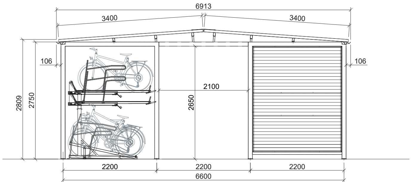
Ansicht von vorne mit Schiebetür
