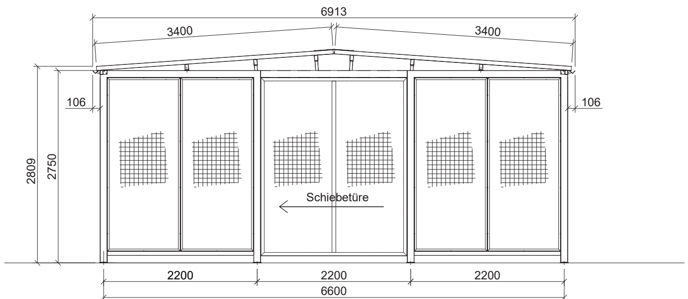
Ansicht von vorne mit Schiebetür
