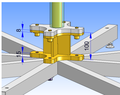
Adapterkonstruktion für extra lange Velos
